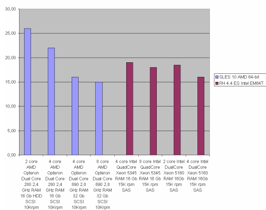
Рис. 3. Результаты тестирования ANSYS на мощных серверах
