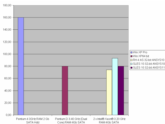
Рис. 2. Результаты тестирования ANSYS для рабочих станций и сервера начального уровня
